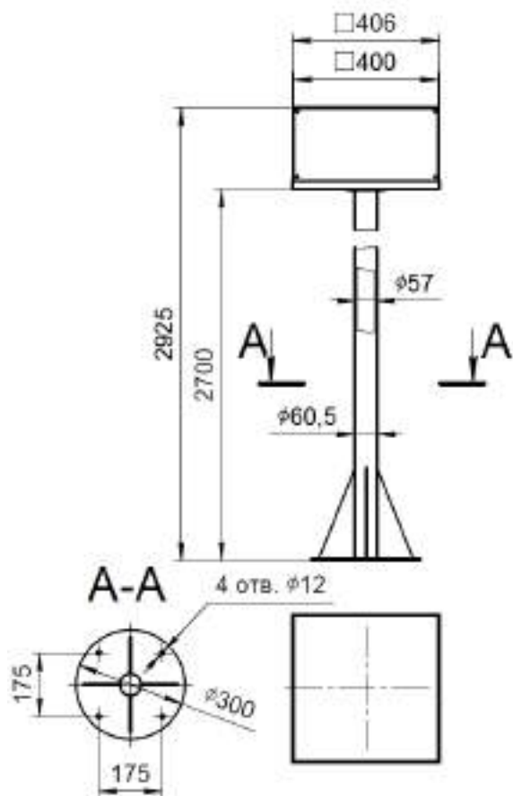
Рис. №2 Габаритный чертёж.
